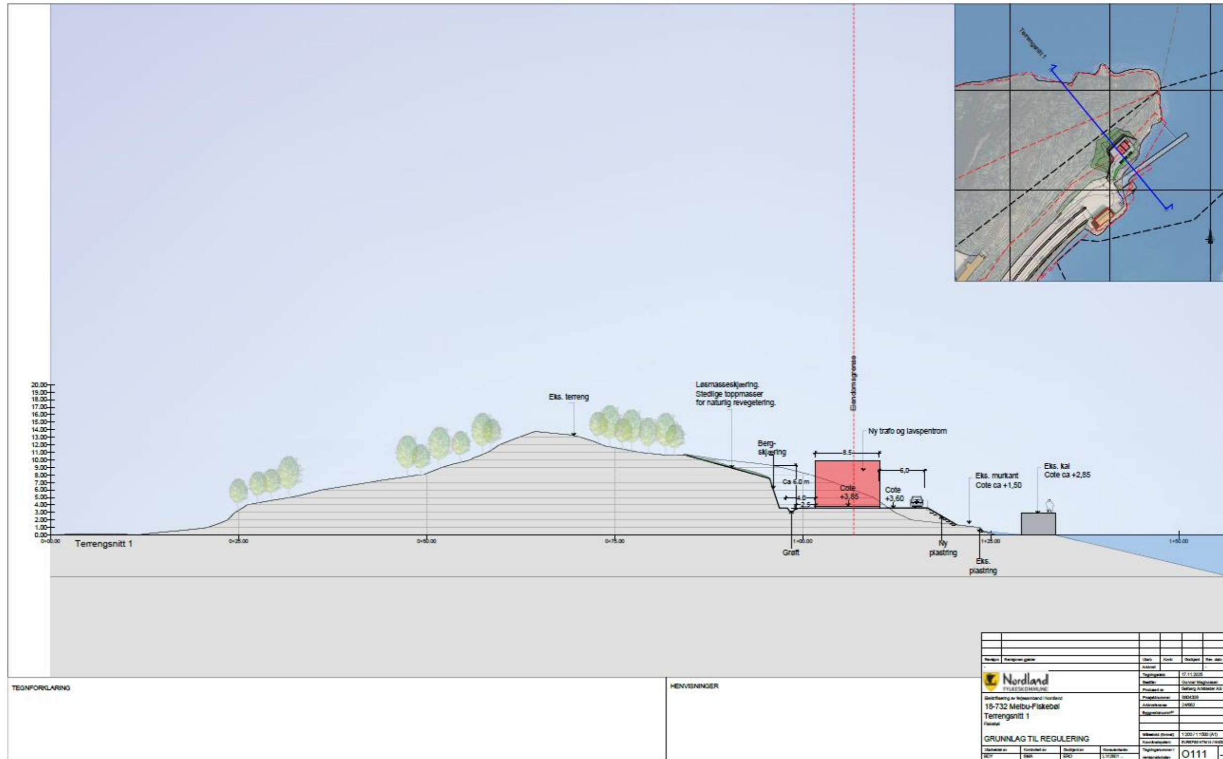
Figur 2. Terrangsnitt 1
